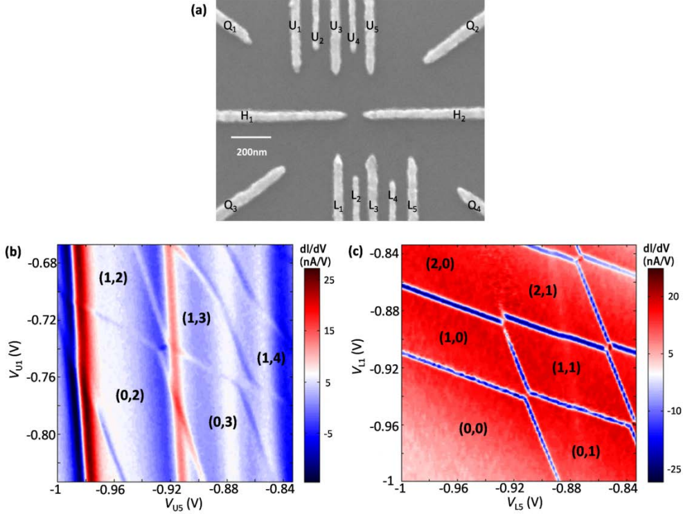
图 4.2 (a)我们的两电荷比特量子点样品 SEM 结构图。(b)和(c)分别为上面和下面双量子点的蜂窝图， (M,N) 代表每个量子点中电荷的填充数目。图片引自文献[9]
