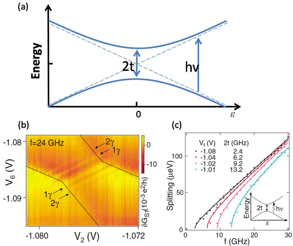
图 3.3 (a)二能级体系对应的能量与能级失谐关系图。(b)连续微波驱动下的单个和两个光子辅助隧穿图像。(c)不同微波频率与一阶峰偏离位置关系图。图片引自文献[9]
